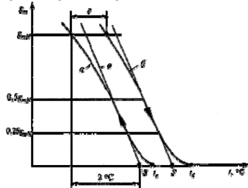
Кривые открытия и закрытия клапана
