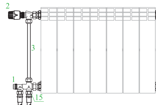
УЗЕЛ "Б"
