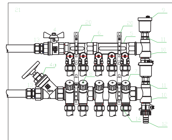
УЗЕЛ "Б"
